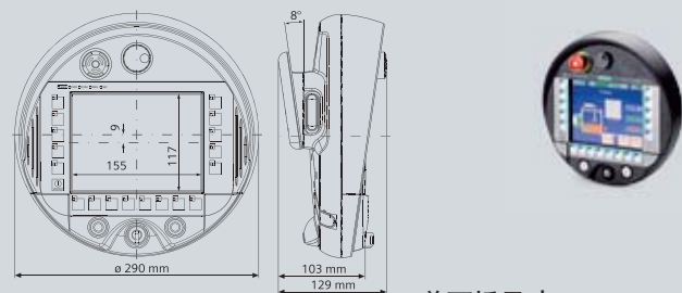
移动面板 277F IWLAN V2
