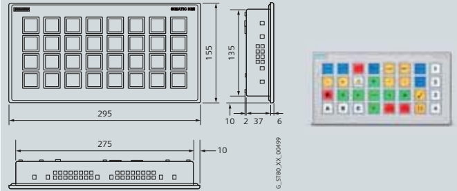
KP32F PN 按键面板
