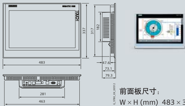
TP1900 精智面板
