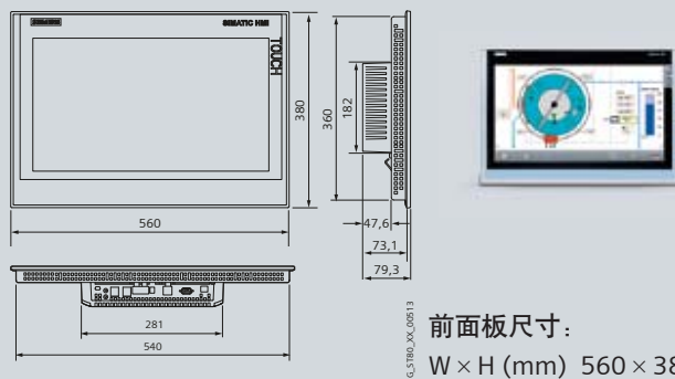
TP2200 精智面板
