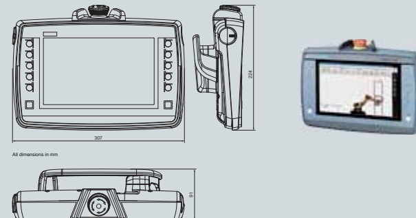
KTP900F 第二代移动面板
